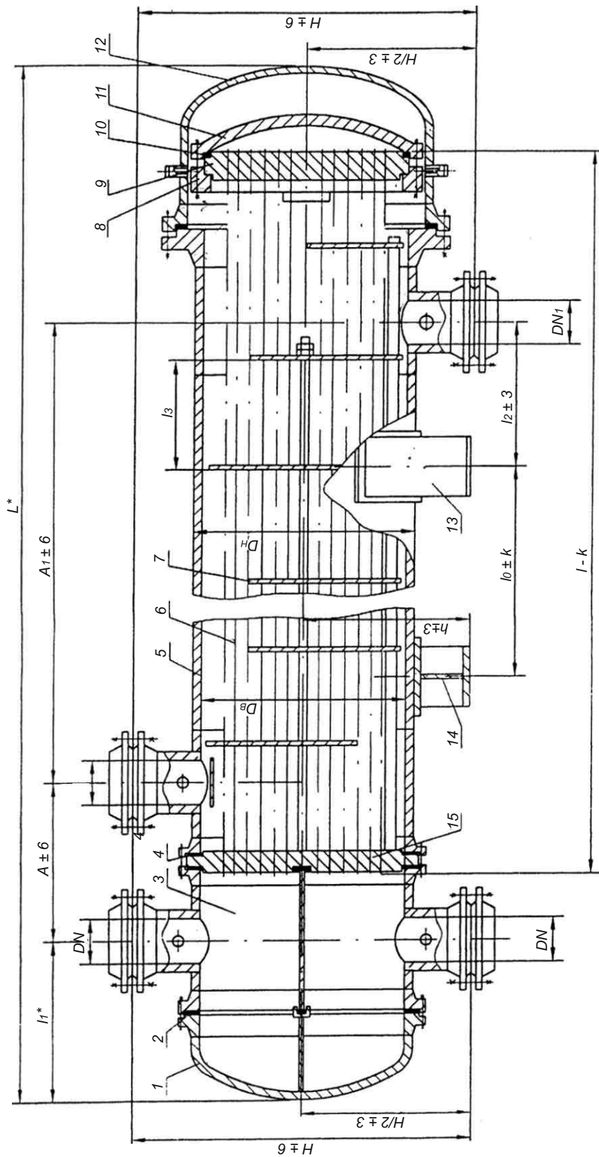
Аппарат типа ТПГ
